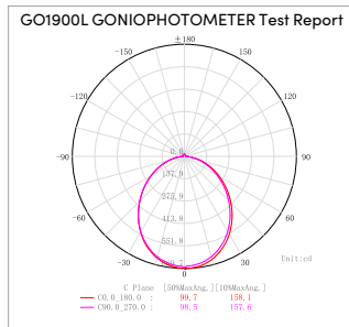
20W-100°-3000K
